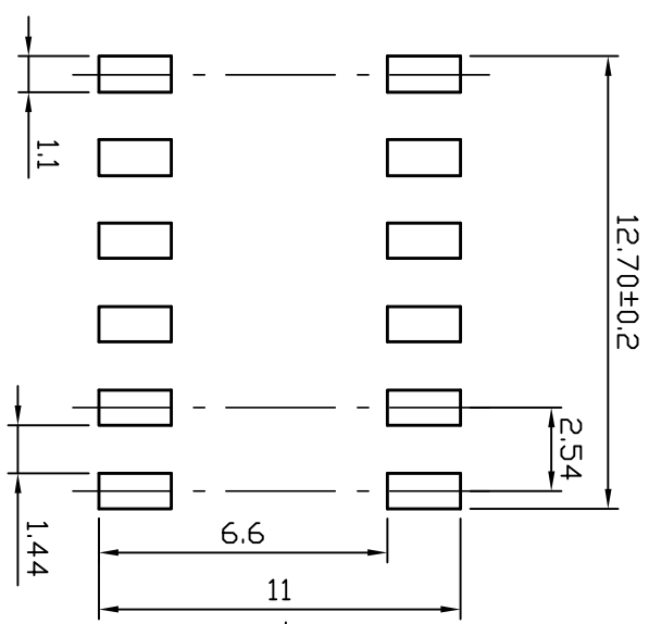
P.C.B LAYOUT
