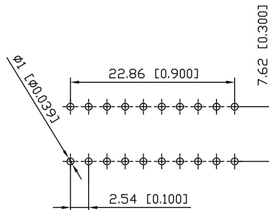
P.C.B LAYOUT
