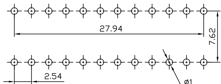
P.C.B LAYOUT
