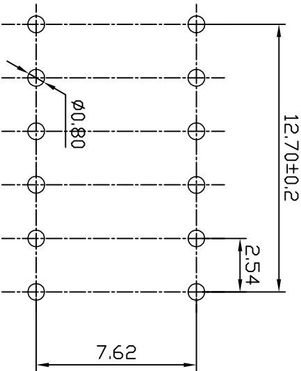
P.C.B LAYOUT
