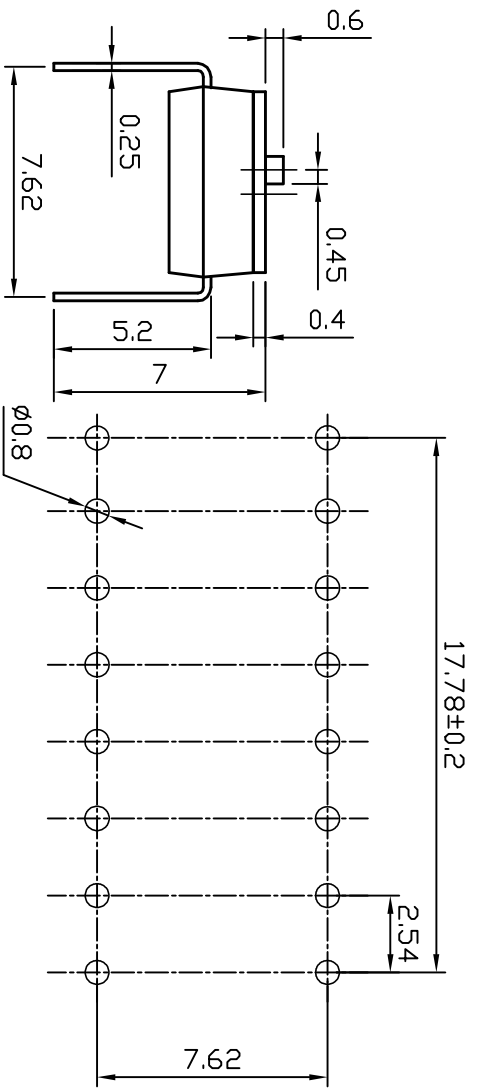
P.C.B LAYOUT
